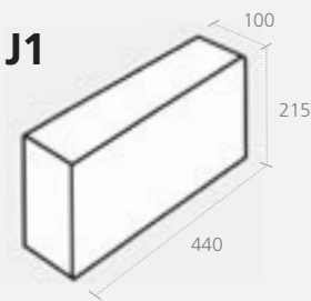
Plain Plinth
